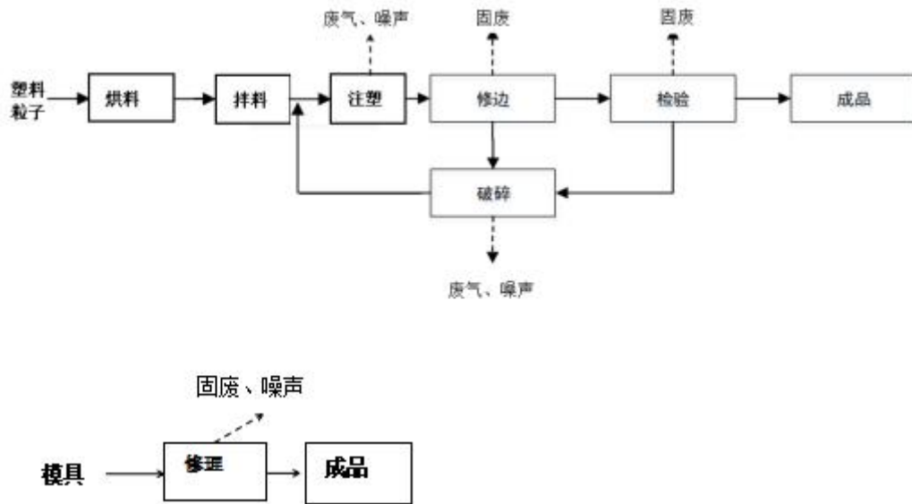
图 2-1 本项目工艺流程及产污环节
