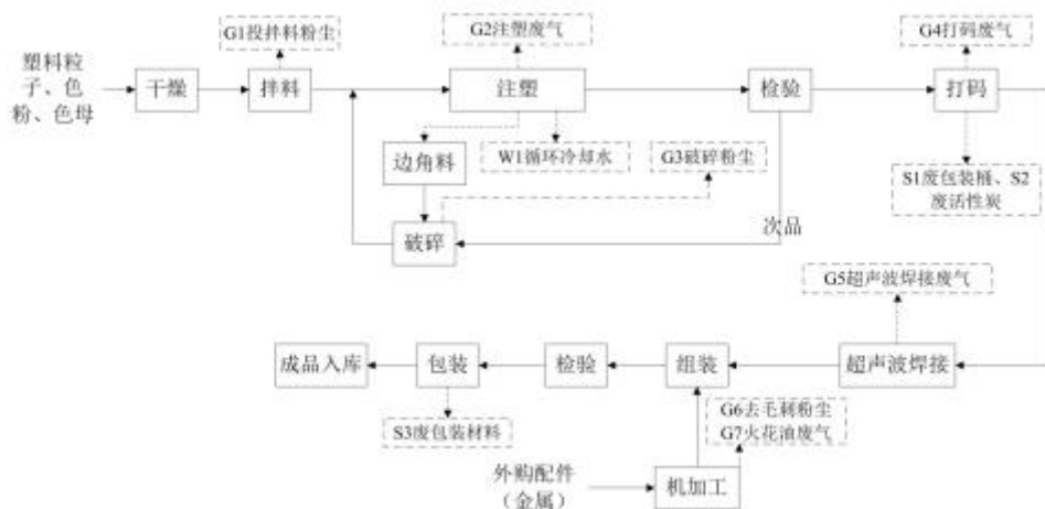
图 2-1 本项目工艺流程及产污环节
