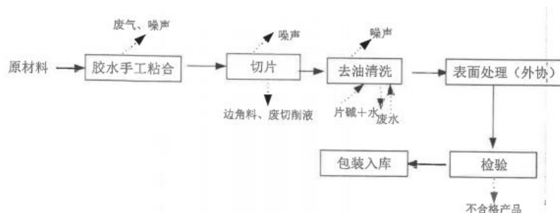
图 2-1 本项目工艺流程及产污环节
