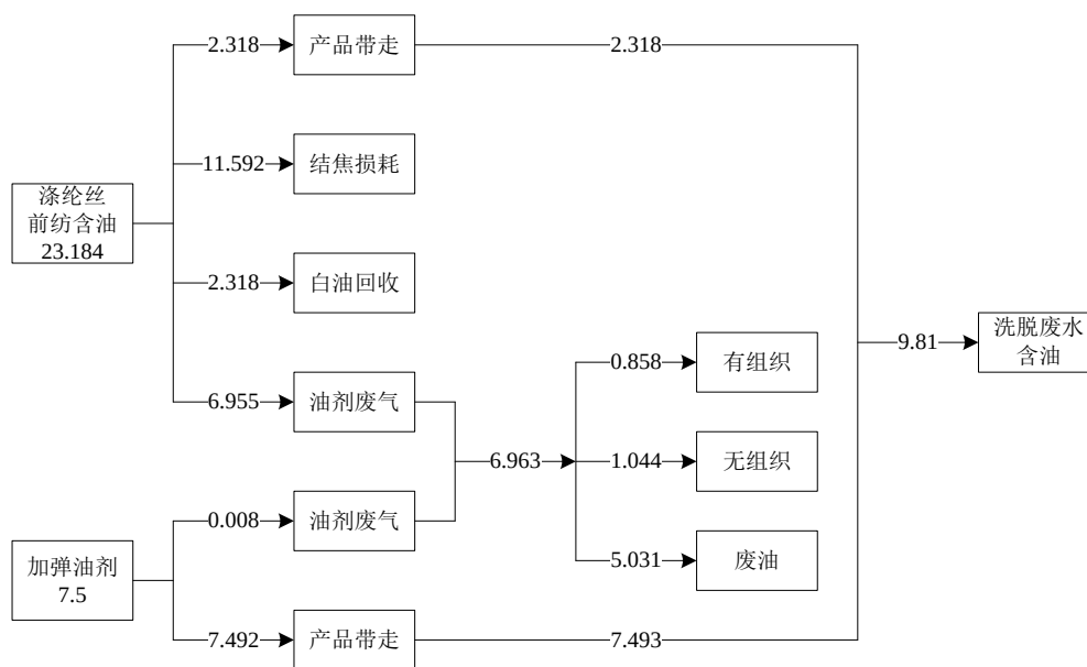
图 3.1-4 油剂平衡图 (1) ——加弹 单位: t/a
