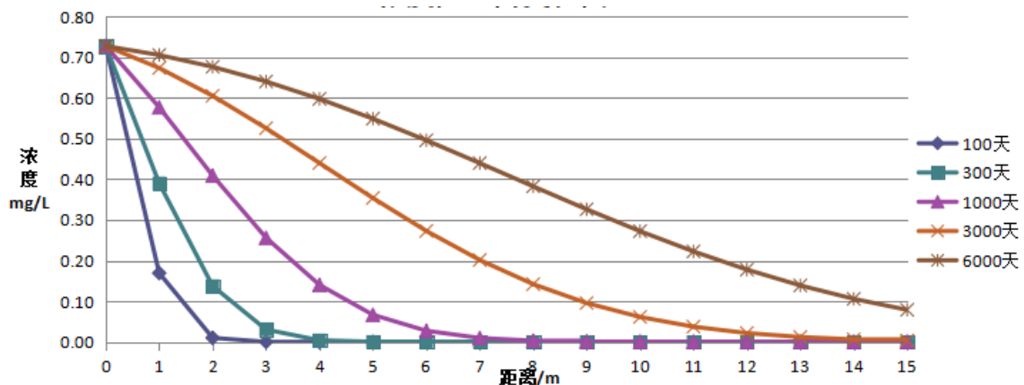
图5.2-1 固定时间不同距离地下水影响预测结果 (总铅)
