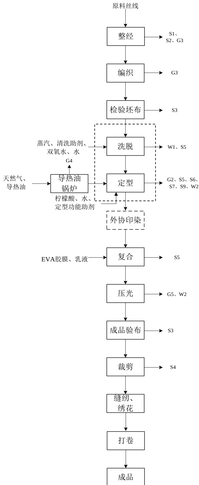
图 3.1-3 梭织布料生产工艺流程及产污节点图
