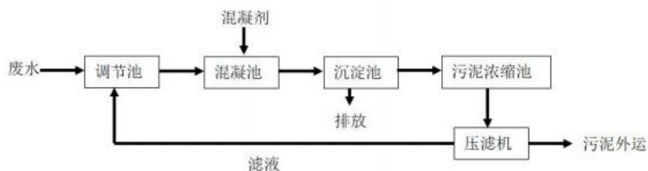
图3-1 废水处理工艺
