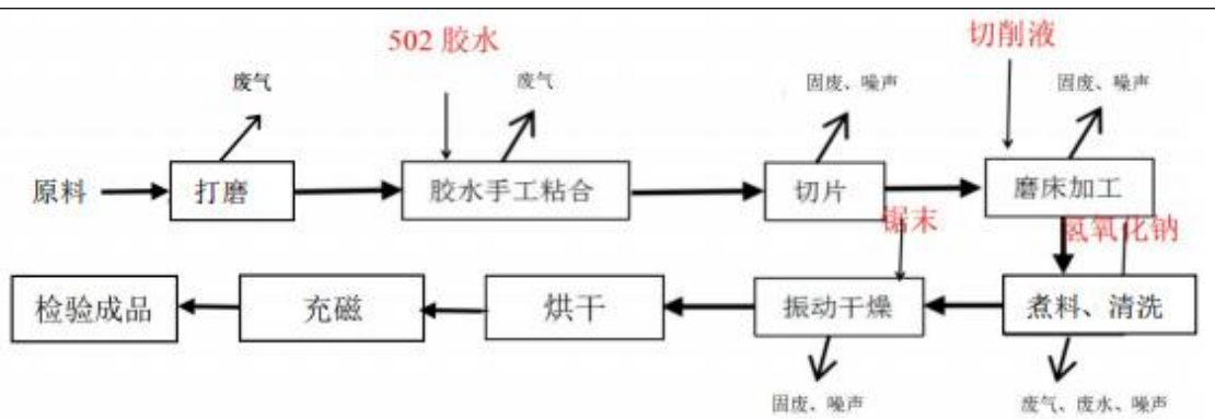
图 2-1 本项目生产工艺流程及产污环节
