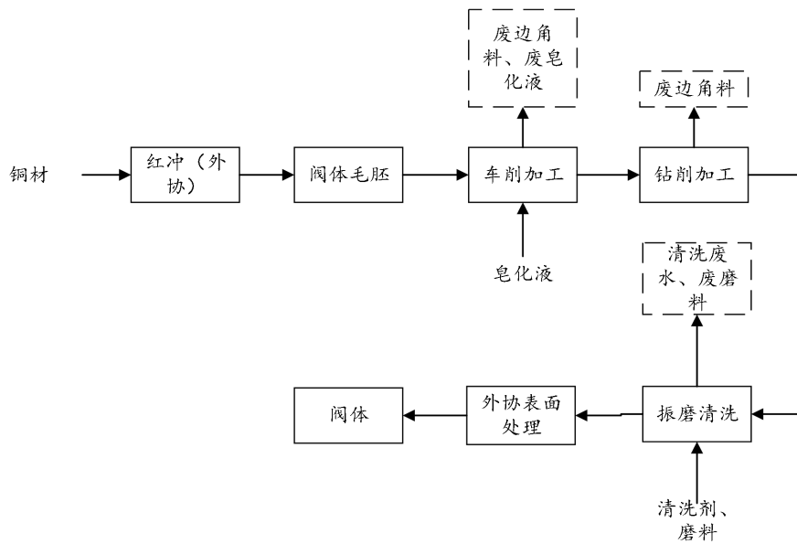
图 2-2 阀体生产工艺流程图
