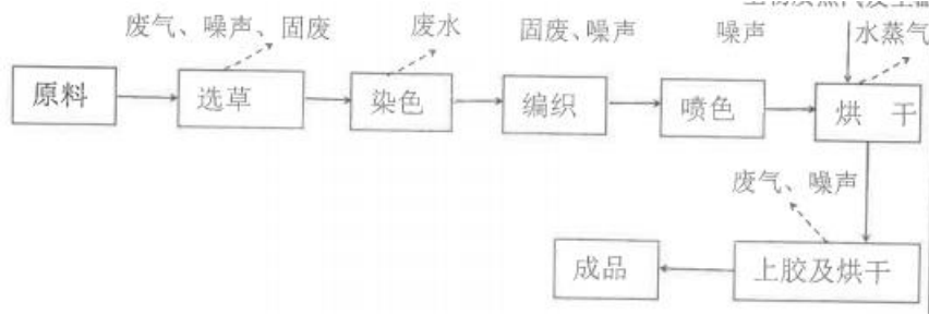
图 2-1 本项目生产工艺总流程及产污环节
