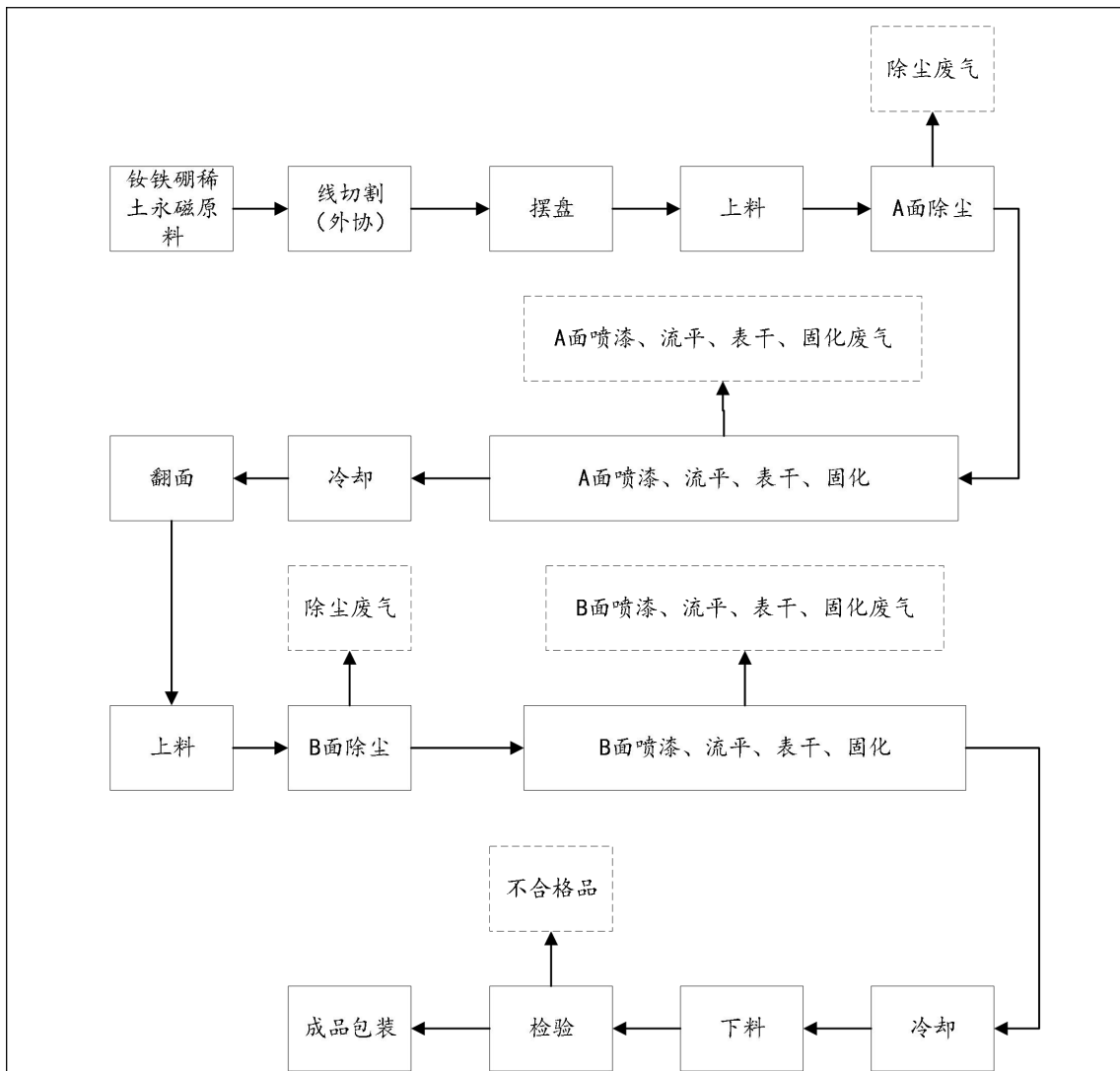
图 2-1 本项目生产工艺总流程及产污环节
