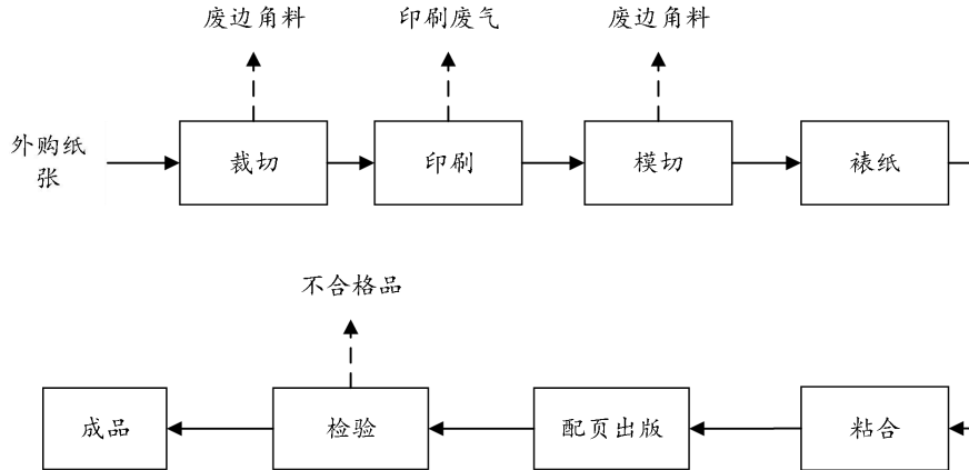
图 2-1 生产工艺及产污节点图
