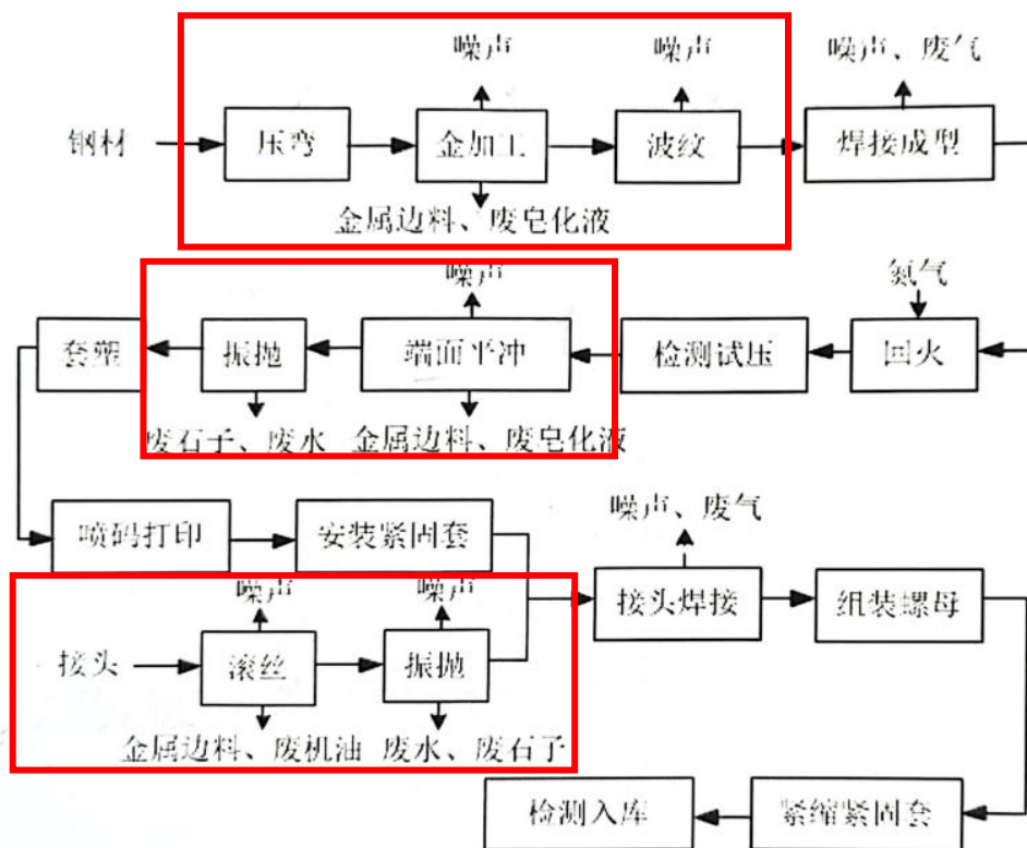
图 2-1 本项目生产工艺总流程及产污环节（红框内生产工序已取消，其中端面平冲改成冲平工序，取消外购接头直接改成铜棒机加工成接头）
