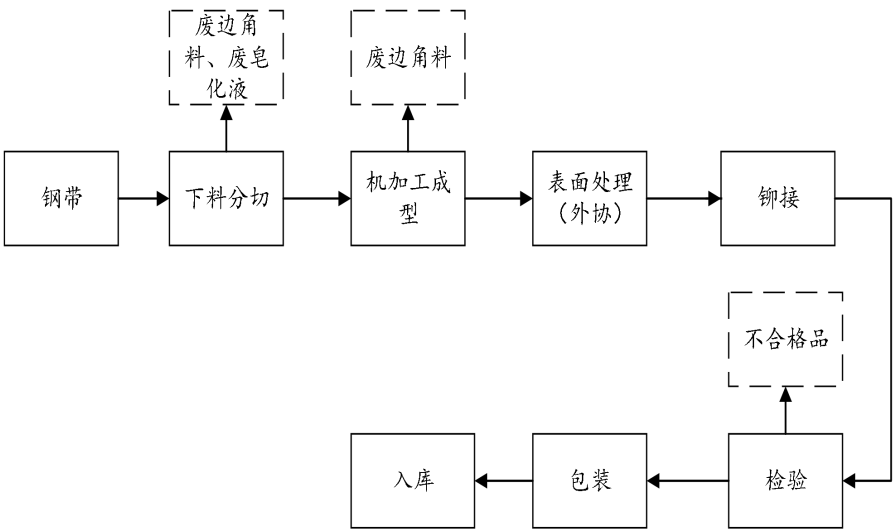
图 2-1 铰链生产工艺及产污节点图
