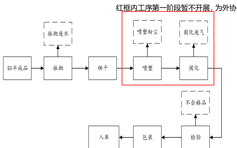
图 2-2 把手生产工艺及产污节点图
