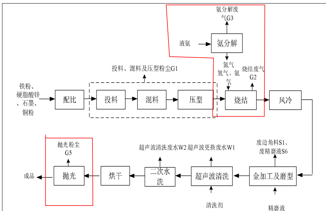
图 2-1 粉末冶金件生产工艺及产污节点图（红框内工艺本阶段暂未开展，均为外协）
