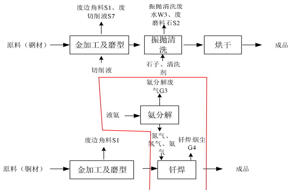
图 2-2 机械配件生产工艺及产污节点图（红框内工艺本阶段暂未开展，均为外协）
