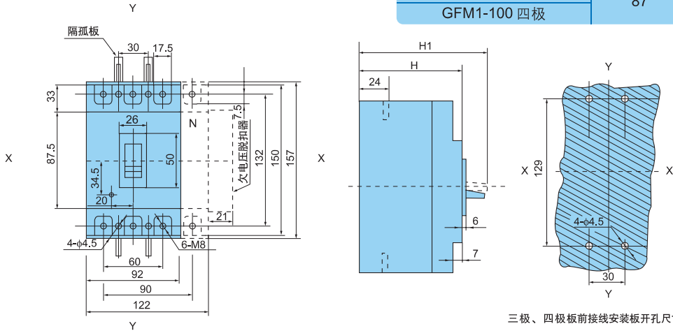
三极、四极板前接线安装板开孔尺寸
