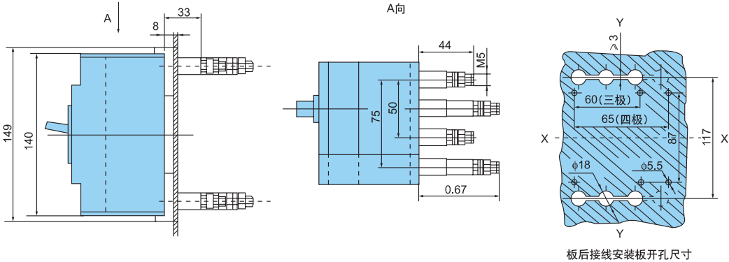
板后接线安装板开孔尺寸
