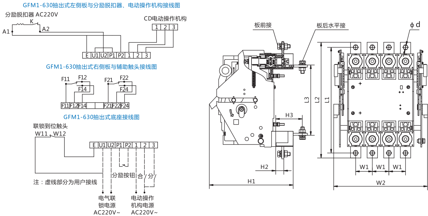
CH2小室后板开孔图及相关尺寸（仅适用于板前出线）
