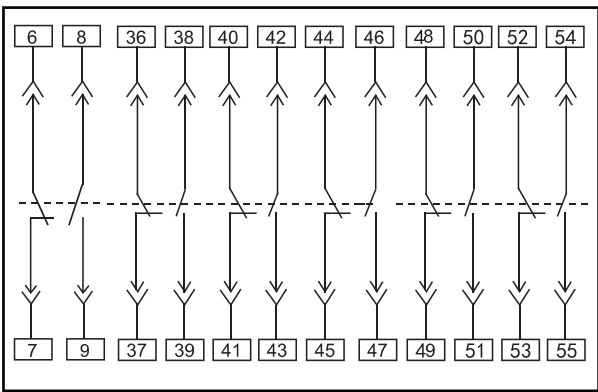
10.4.4 辅助为六常开六常闭在H型控制器的状态下
