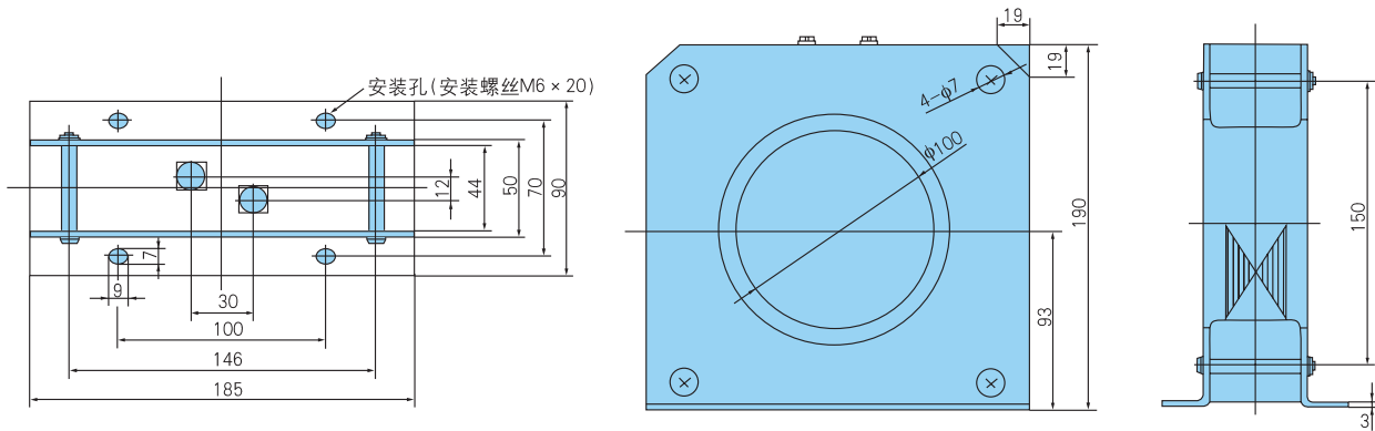
ZT100互感器
