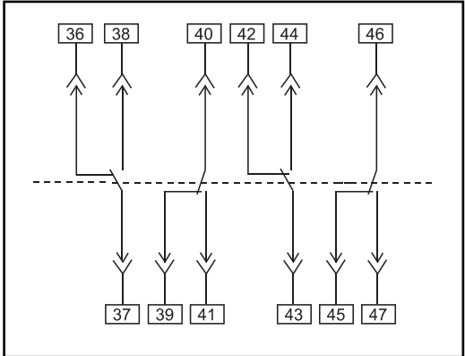
10.4.1 辅助四组为转换触头（常规发货）
