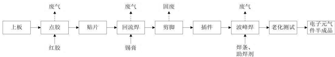
图 2-3 电子元器件生产工艺流程图
