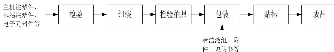
图 2-4 组装工艺流程图
