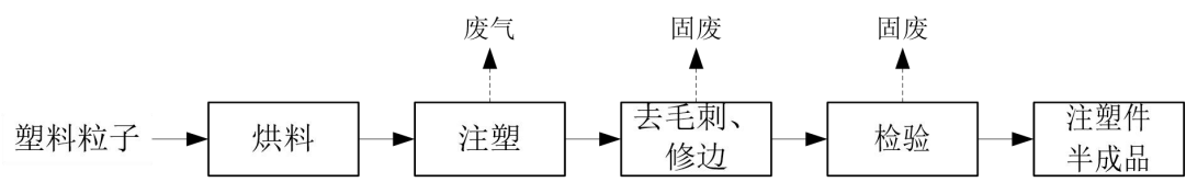
图 2-2 项目生产工艺流程及产污节点图
