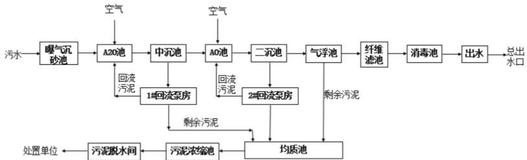
图 4-1 一期工程 30 万 m³/d 生活污水处理工艺流程图
