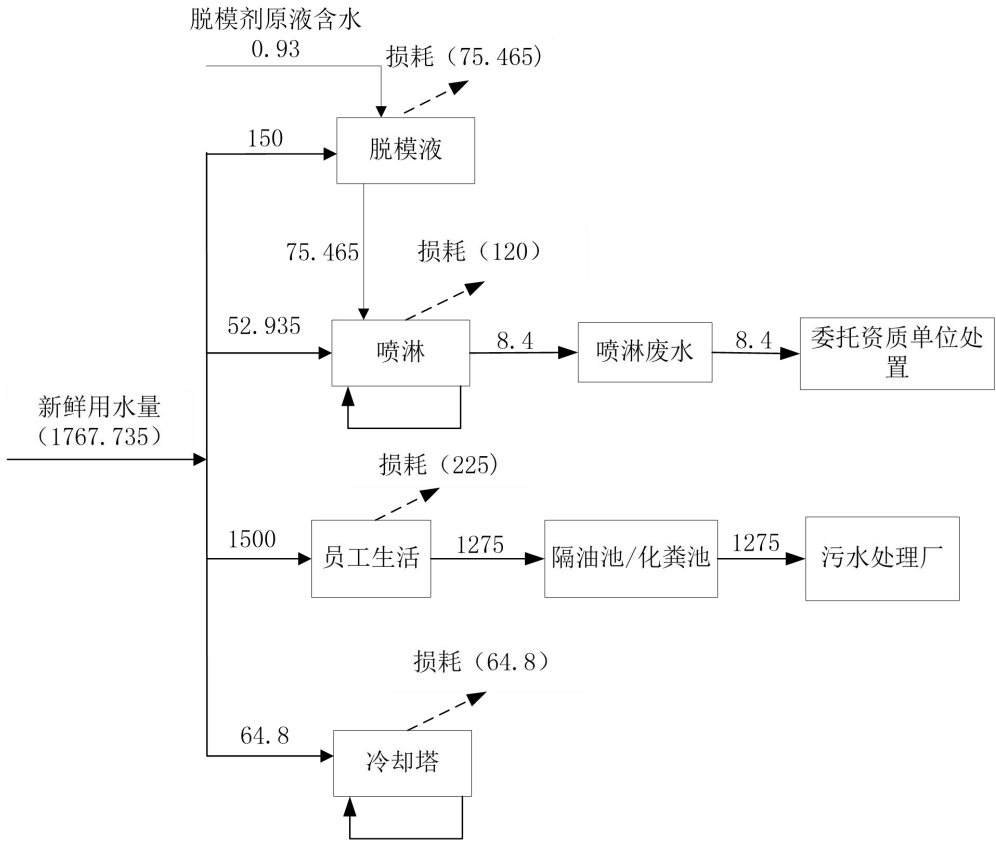
图 2-1 本项目水平衡图
