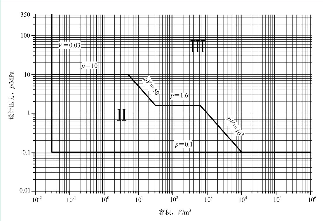
图 A-1 压力容器分类图——第一组介质
