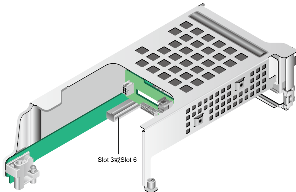
图 5-23 PCIe Riser 卡 2
