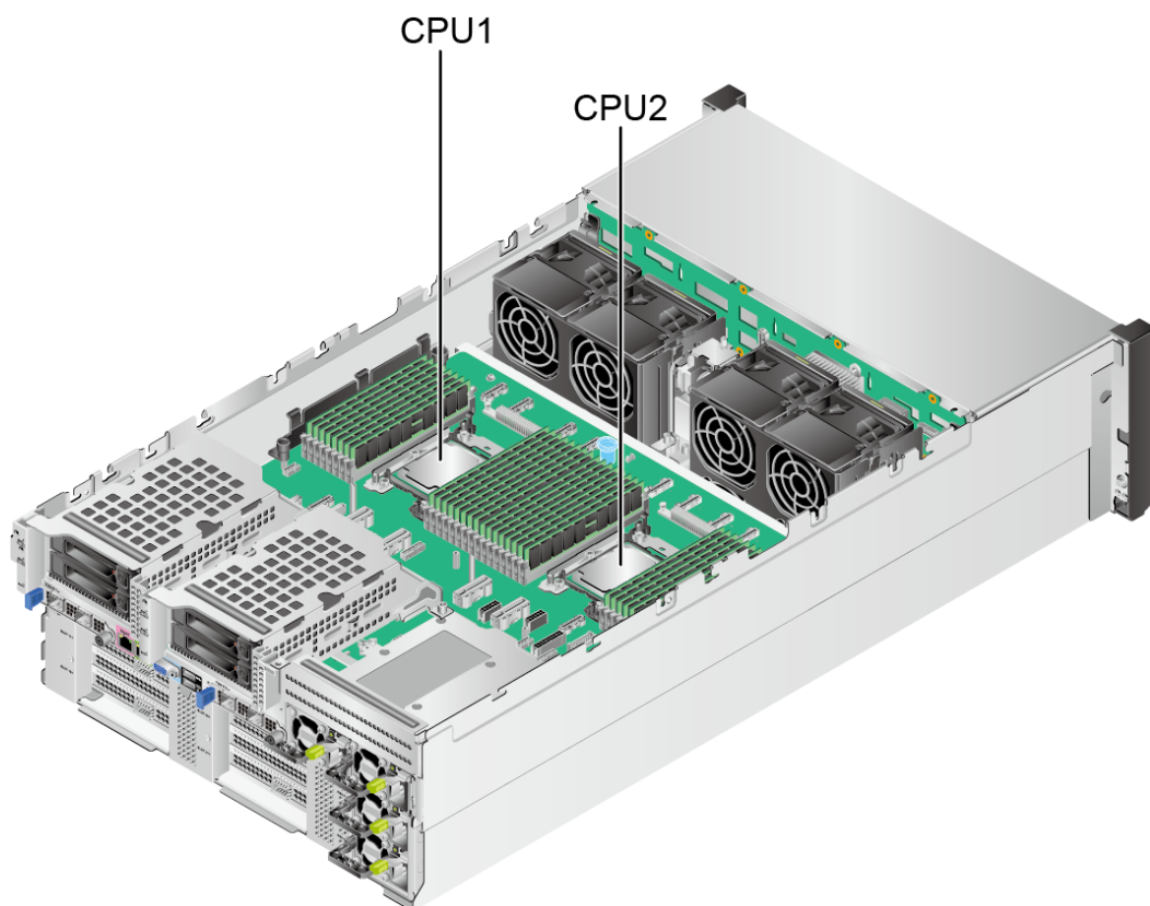
图 5-7 处理器位置
