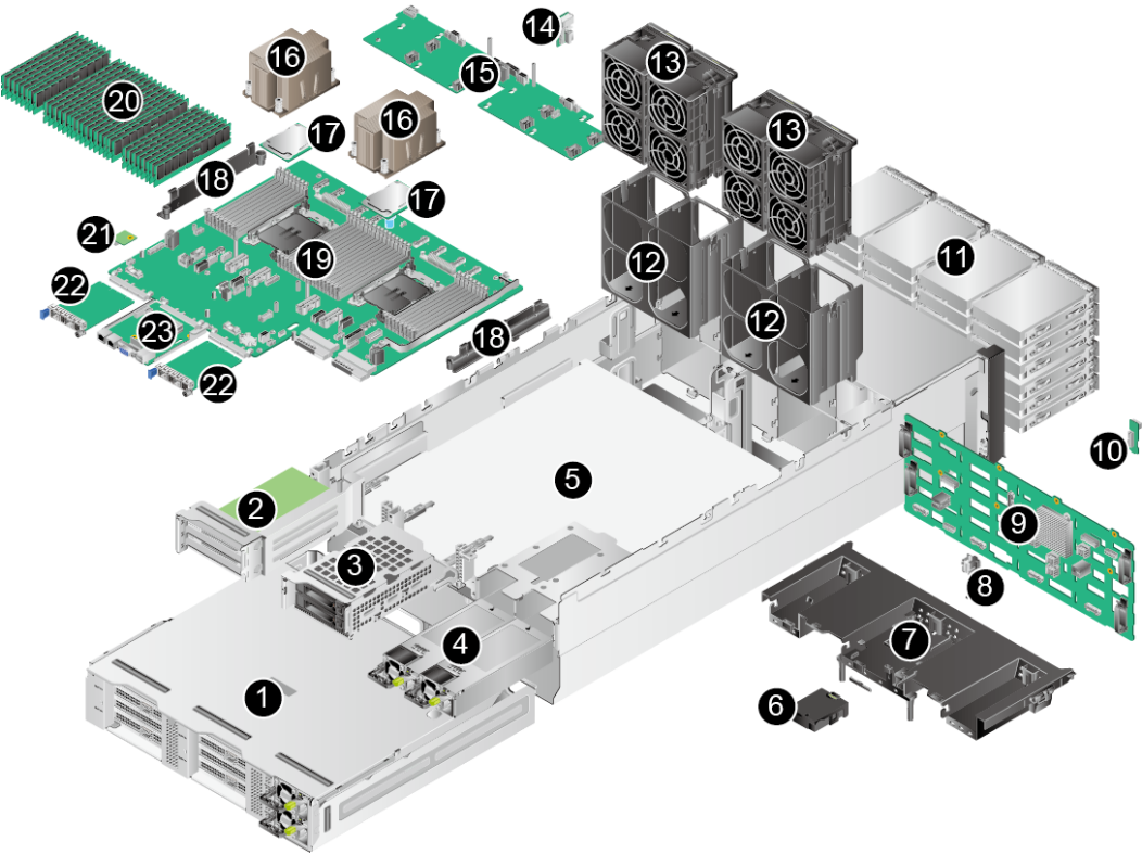
图 3-1 物理结构
