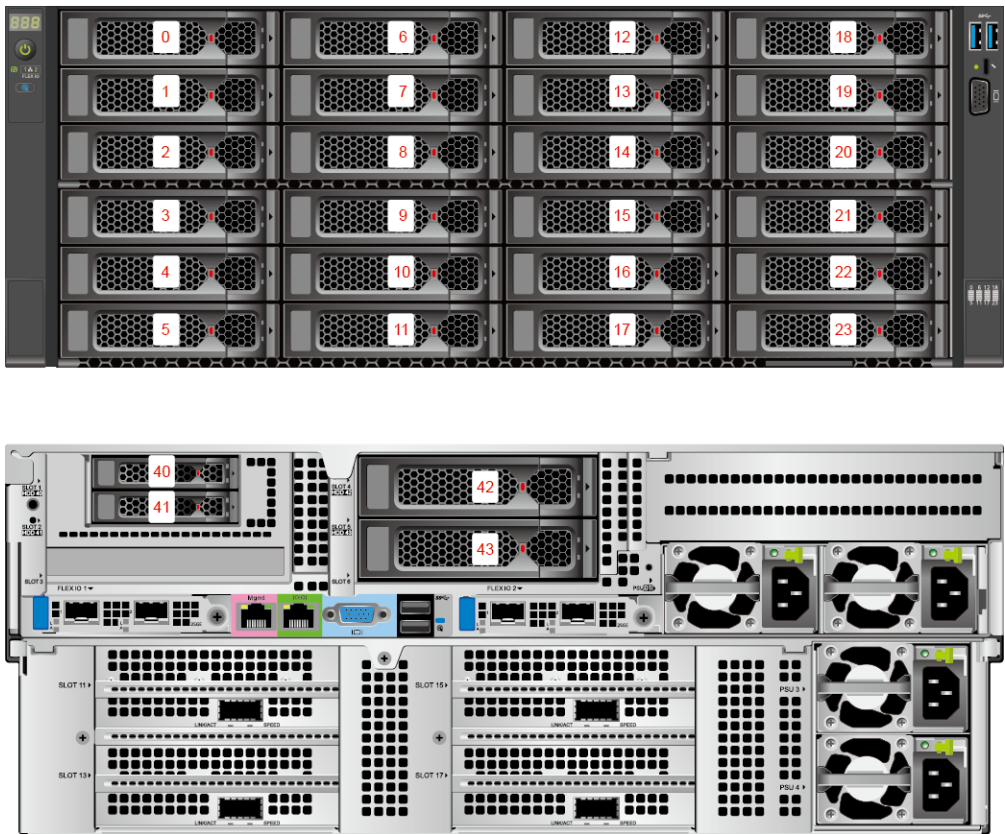
图 5-19 硬盘编号（IO 模组 1 配置 2.5 英寸硬盘+IO 模组 2 配置 3.5 英寸硬盘）
