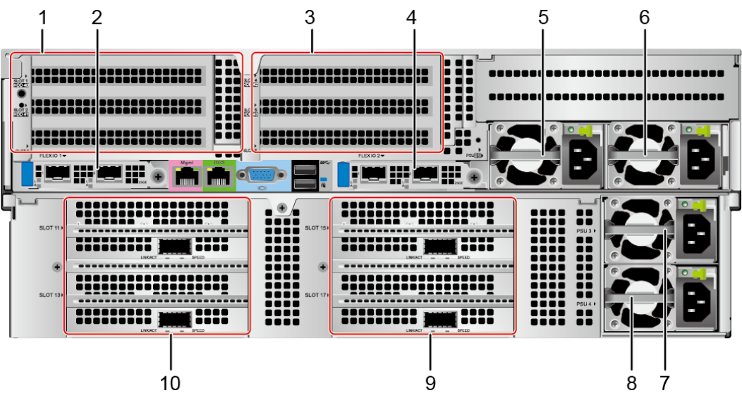
图 5-4 后面板外观
