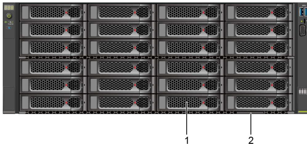
图 5-1 前面板外观
