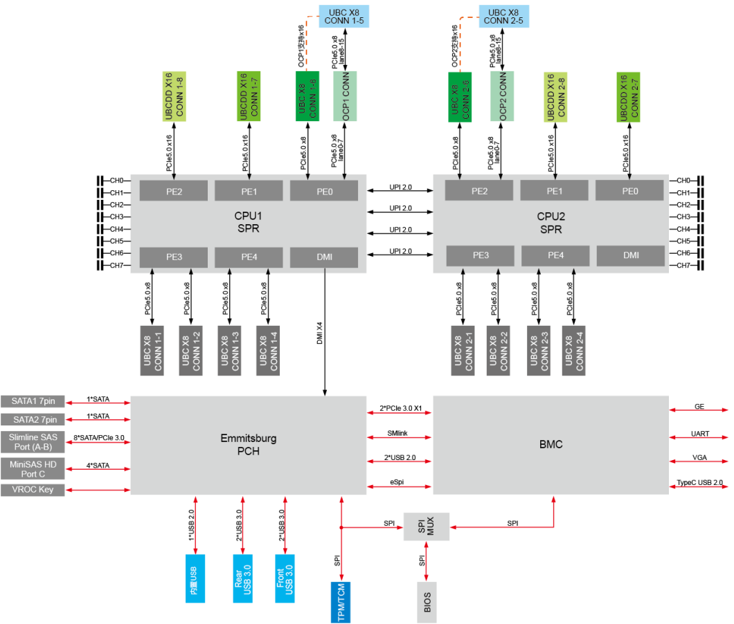
图 4-1 逻辑结构
