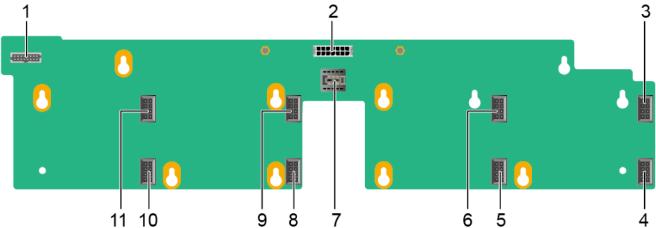
图 5-32 风扇板
