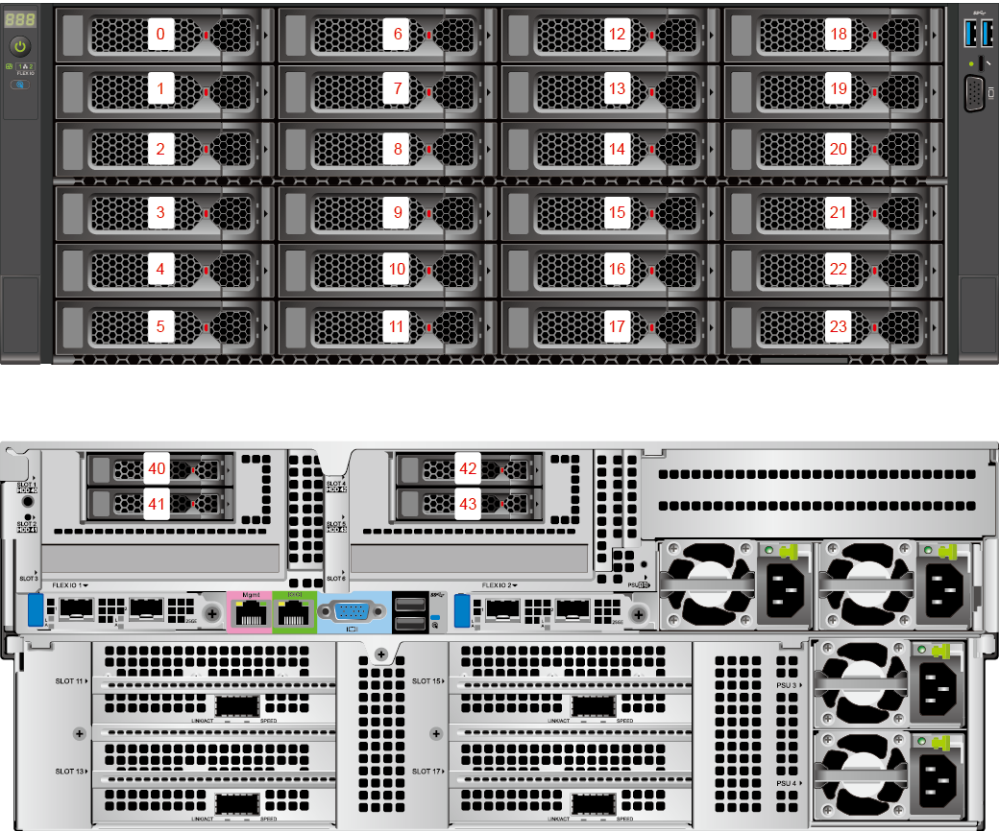
图 5-18 硬盘编号（IO 模组 1 配置 2.5 英寸硬盘+IO 模组 2 配置 2.5 英寸硬盘）
