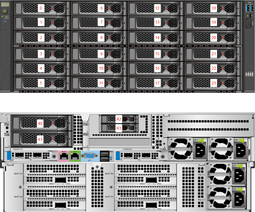
图 5-14 硬盘编号 ( IO 模组 1 配置 3.5 英寸硬盘+IO 模组 2 配置 2.5 英寸硬盘 )
