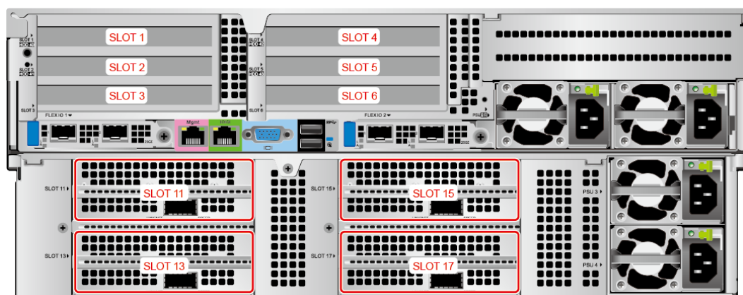
图 5-21 PCIe 插槽
