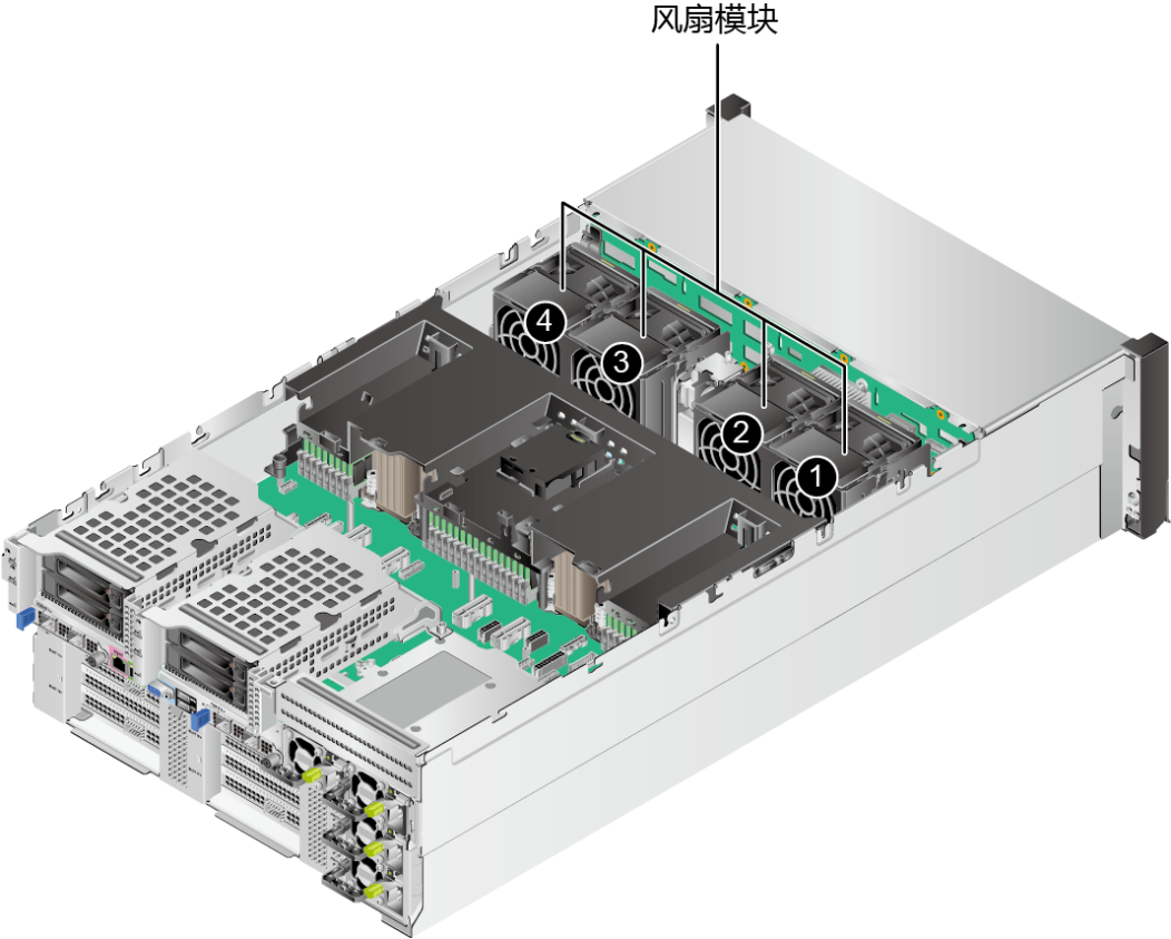
图 5-26 风扇模块的位置
