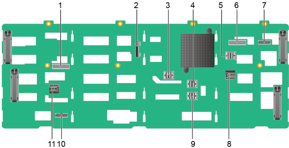
图 5-28 24x3.5 英寸硬盘 EXP 配置背板
