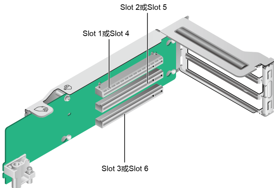
图 5-22 PCIe Riser 卡 1
