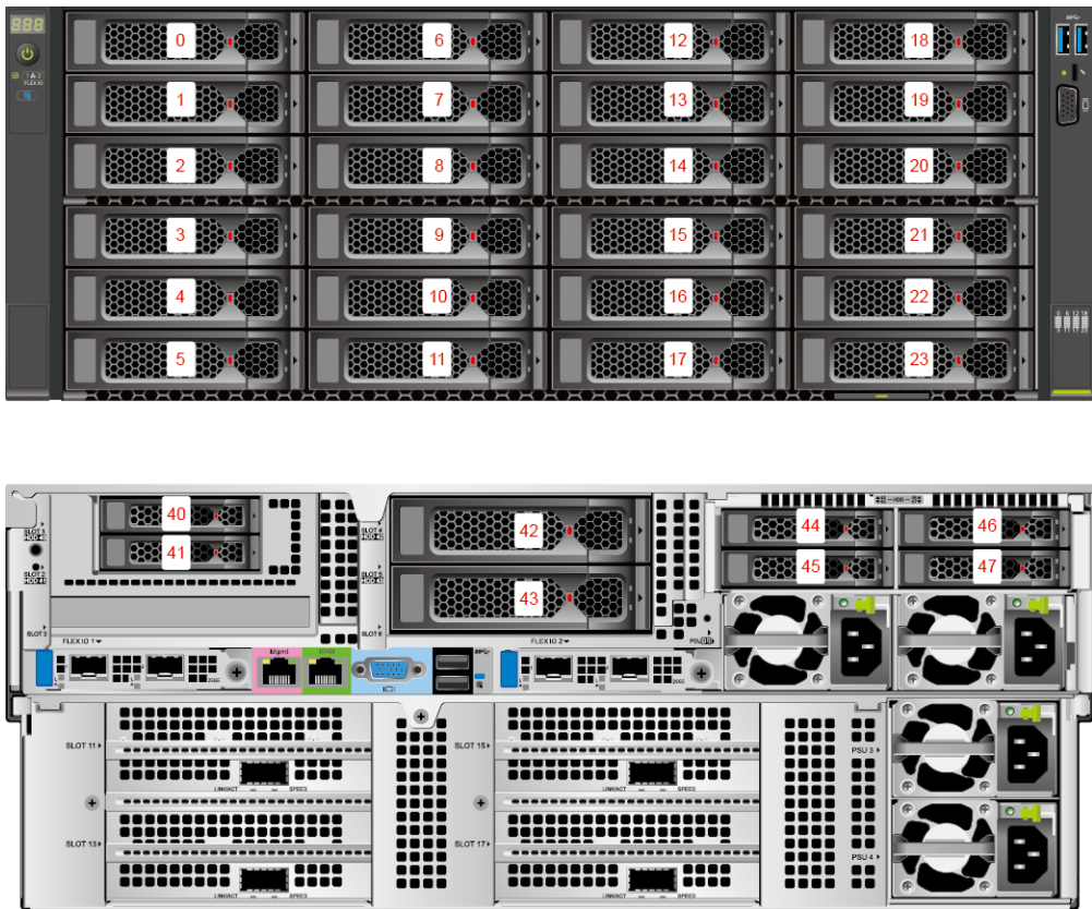
图 5-17 硬盘编号（IO 模组 1 配置 2.5 英寸硬盘+IO 模组 2 配置 3.5 英寸硬盘）
