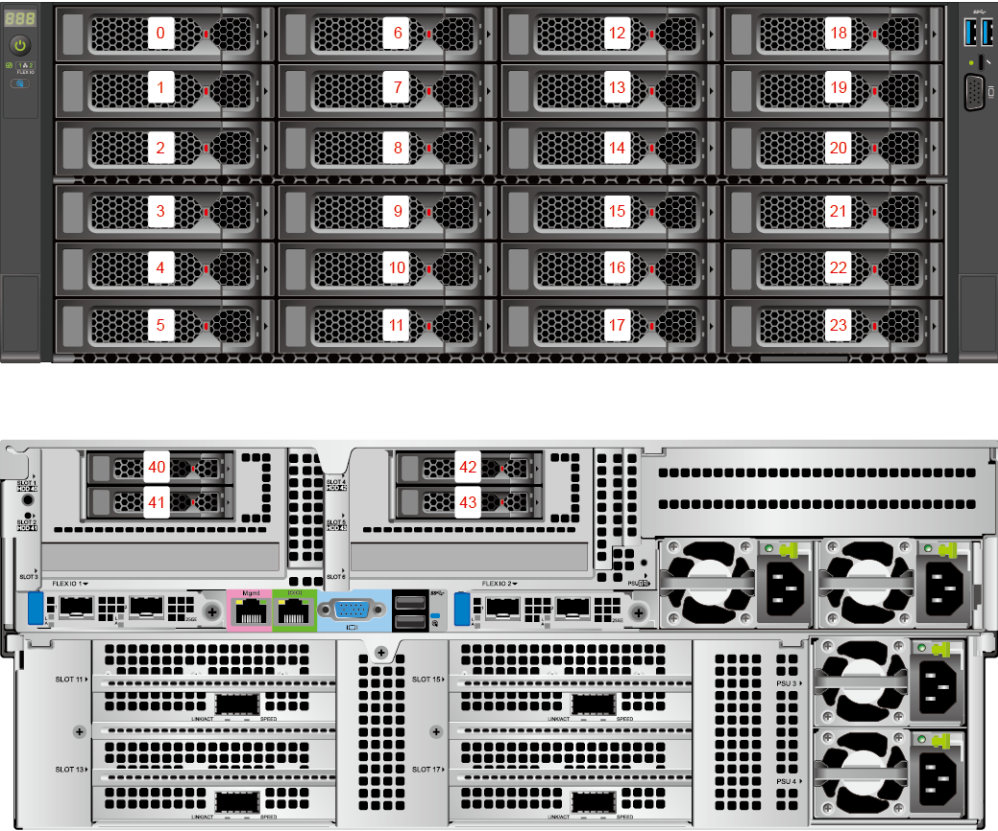
图 5-12 硬盘编号（IO 模组 1 配置 2.5 英寸硬盘+IO 模组 2 配置 2.5 英寸硬盘）
