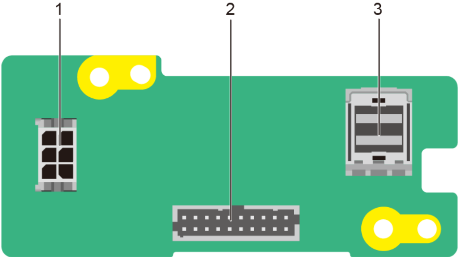
图 5-29 2x2.5 英寸硬盘背板
