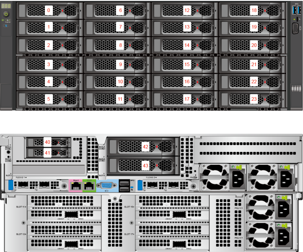
图 5-13 硬盘编号（IO 模组 1 配置 2.5 英寸硬盘+IO 模组 2 配置 3.5 英寸硬盘）
