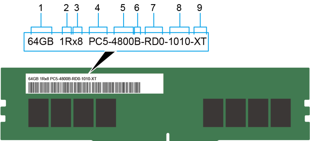
图 5-8 内存标识
