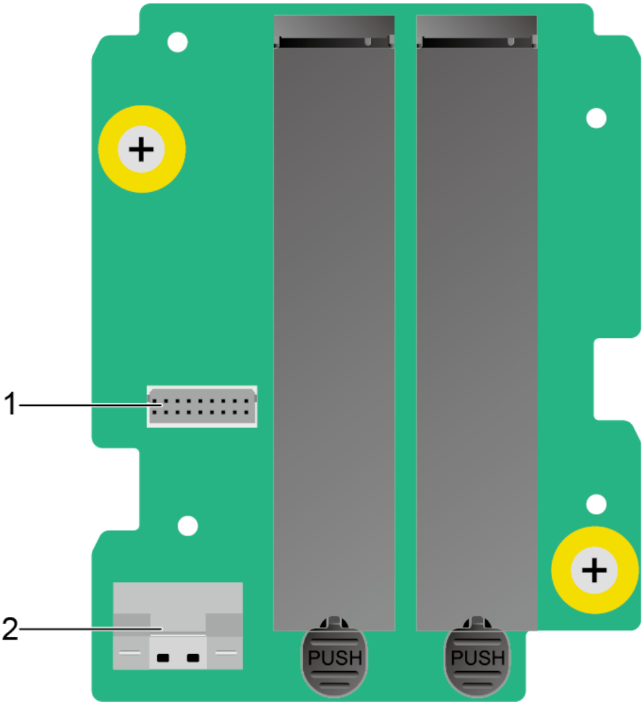
图 5-33 M.2 转接板
