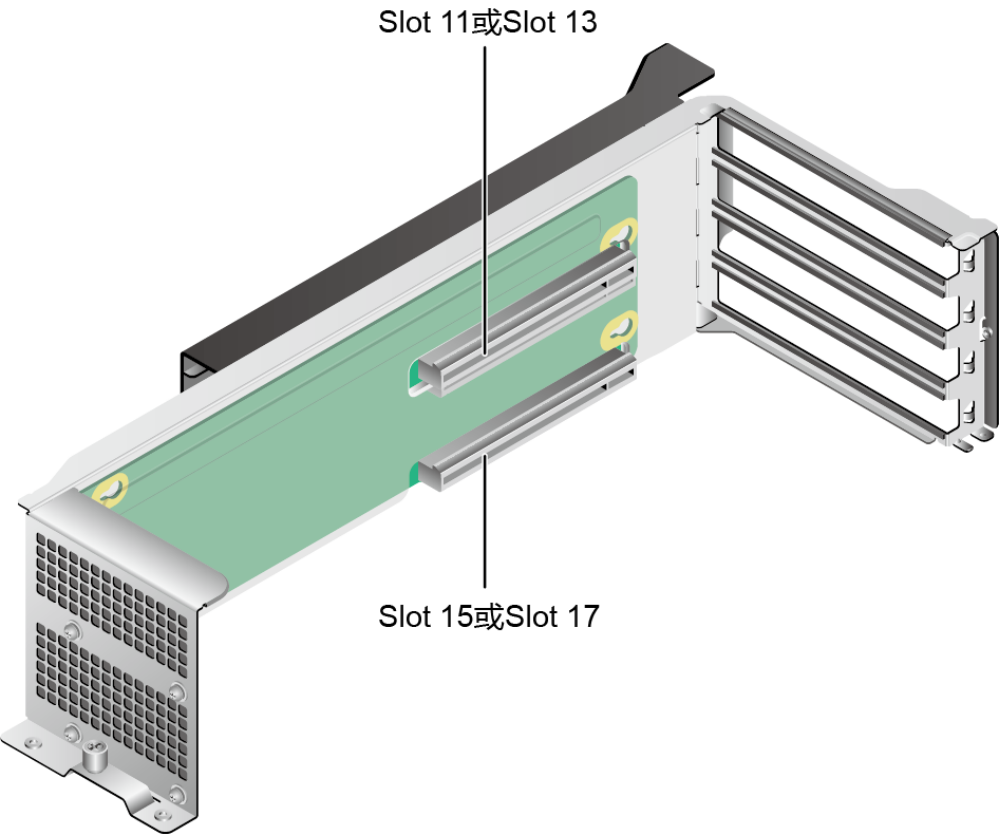
图 5-24 PCIe Riser 卡 ( 电源接口面和 PCIe 槽位面 )
