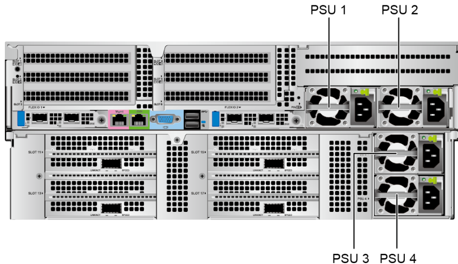
图 5-25 电源模块位置
