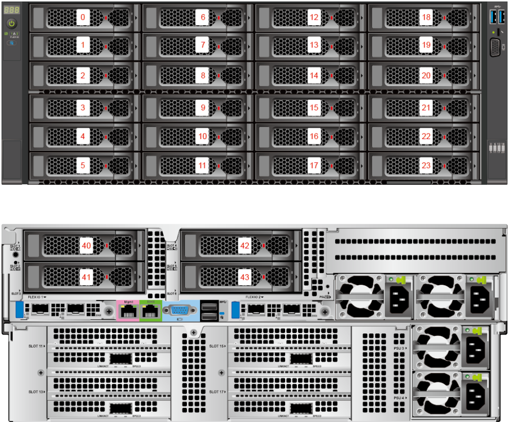
图 5-15 硬盘编号（IO 模组 1 配置 3.5 英寸硬盘+IO 模组 2 配置 3.5 英寸硬盘）
