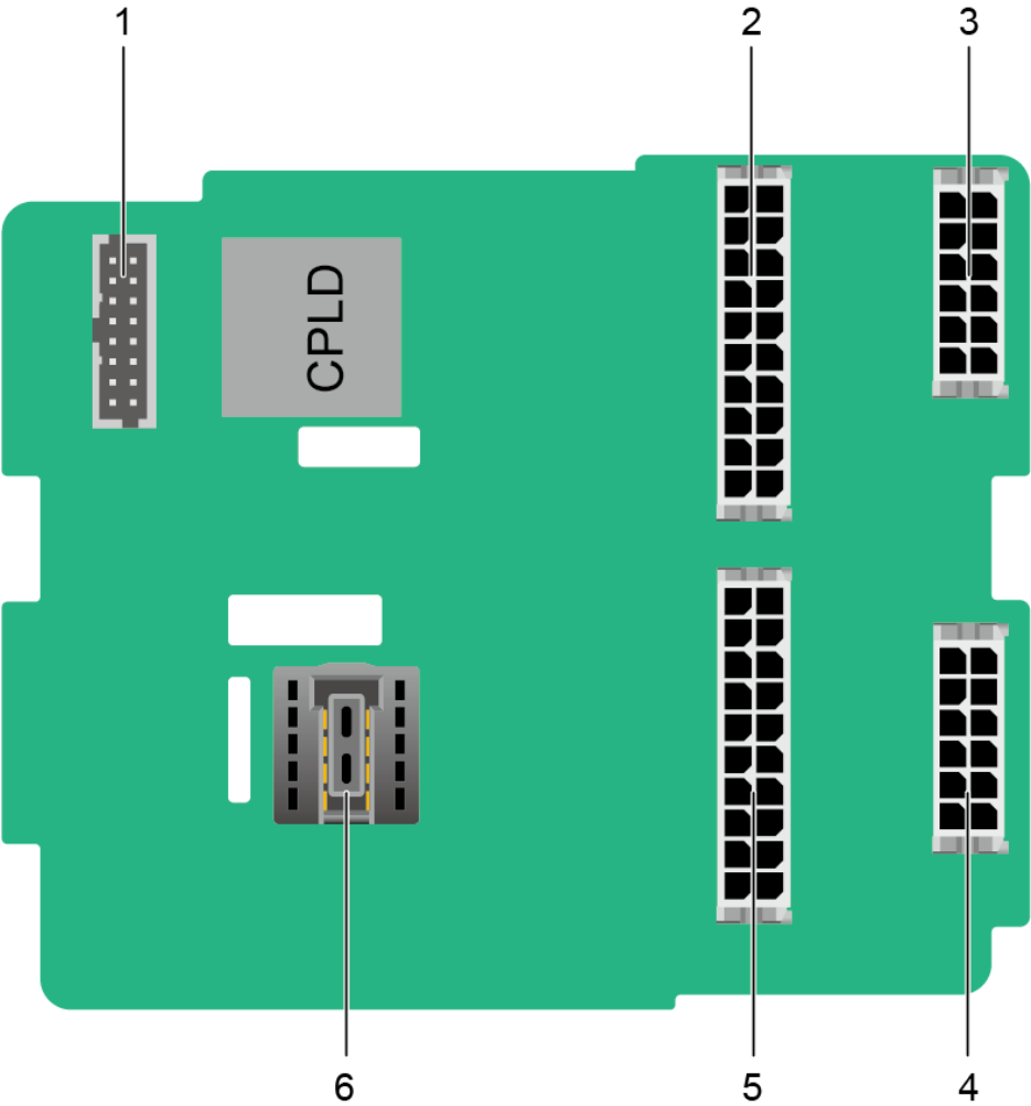
图 5-31 电源背板
