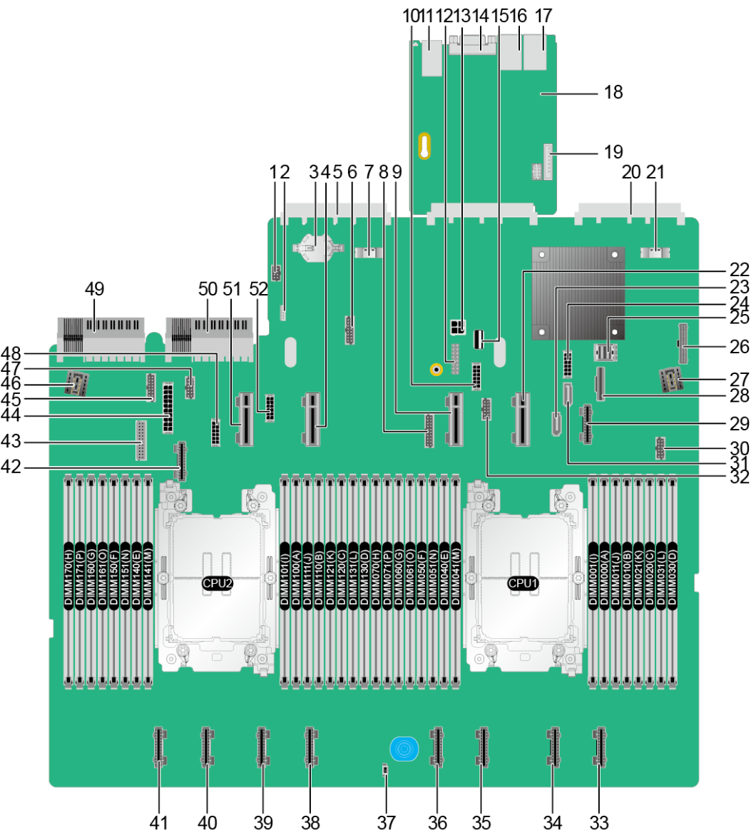
图 5-27 主板
